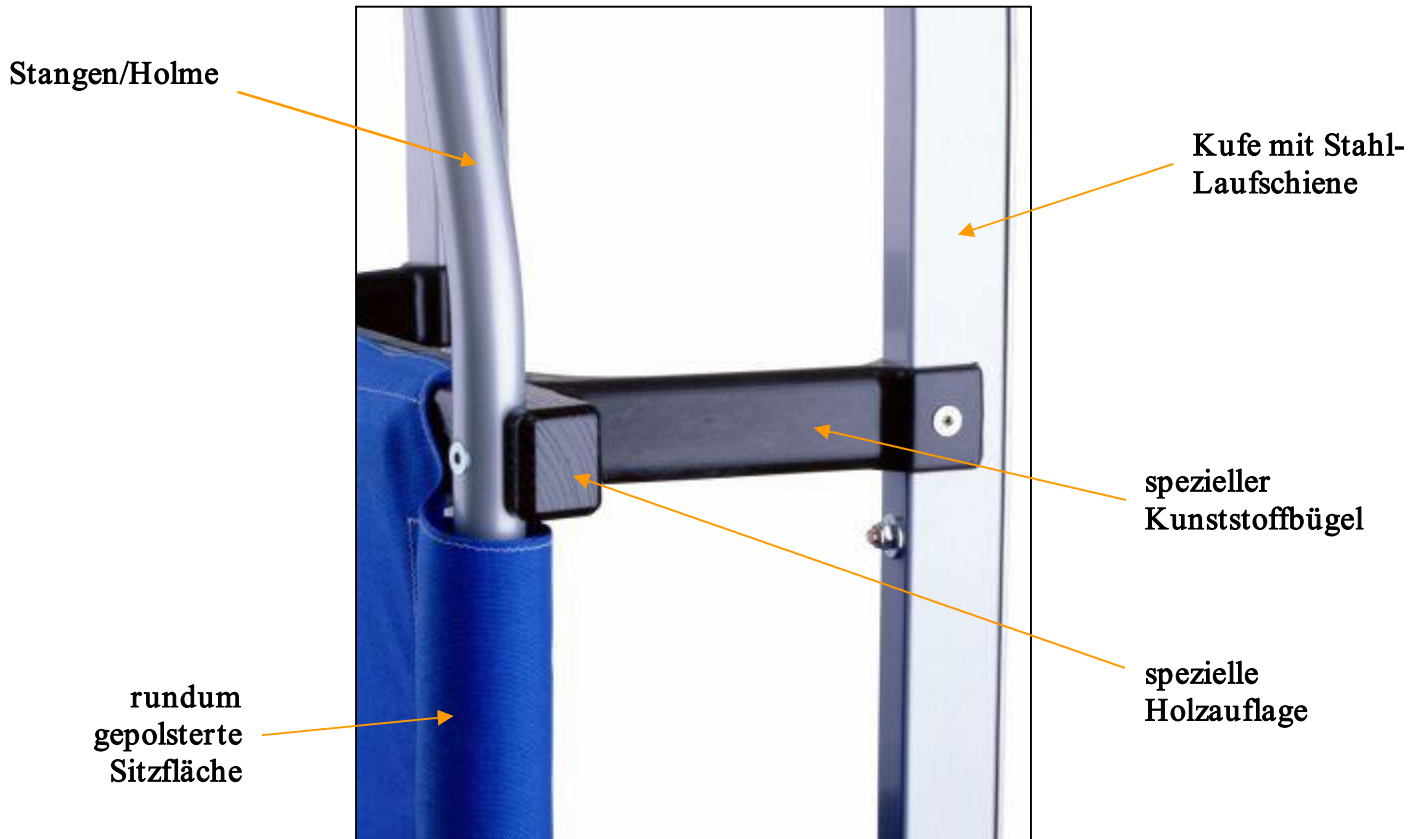
(Detailansicht Kunststoffbankl Alu-K)
